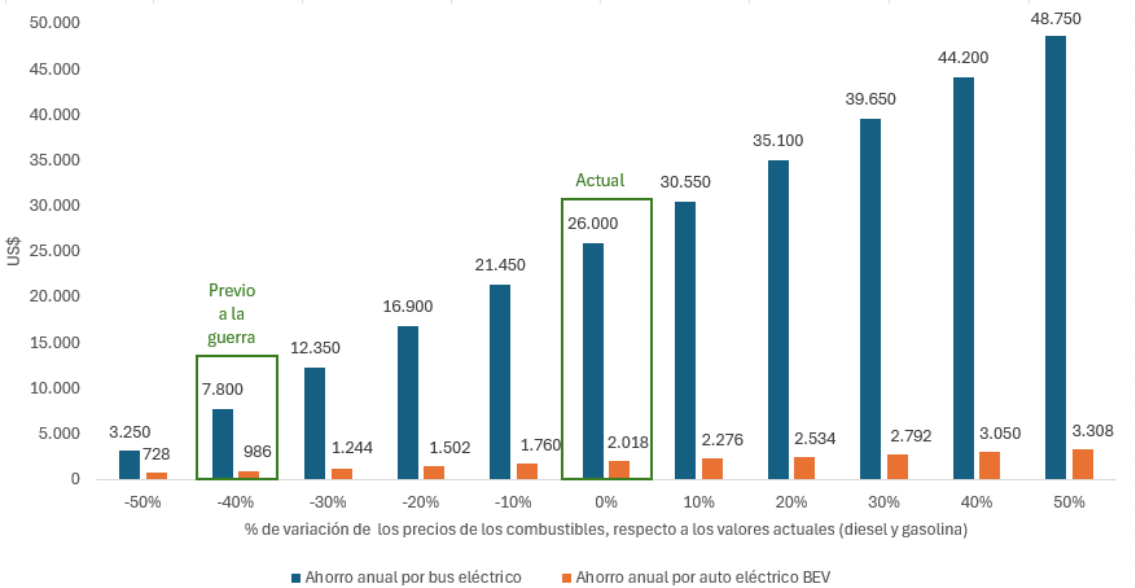
Figura 3. Ahorro económico anual por unidad de vehículo eléctrico, respecto a la variación del precio de los combustibles.
