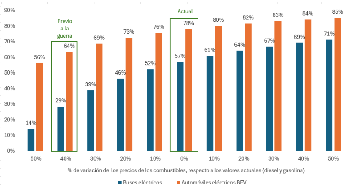
Figura 2. Porcentaje de ahorro económico en energía por km, respecto a la variación del precio de los combustibles.
